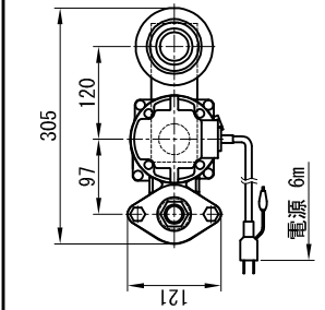
スクレープロボ 上面視
